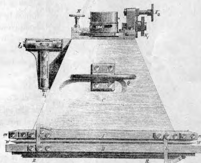
Fig. 3. Cámara; proyeccion horizontal.
